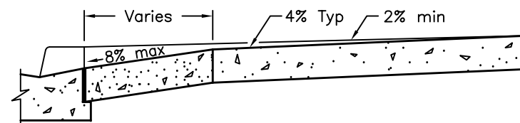
SECTION D-D
